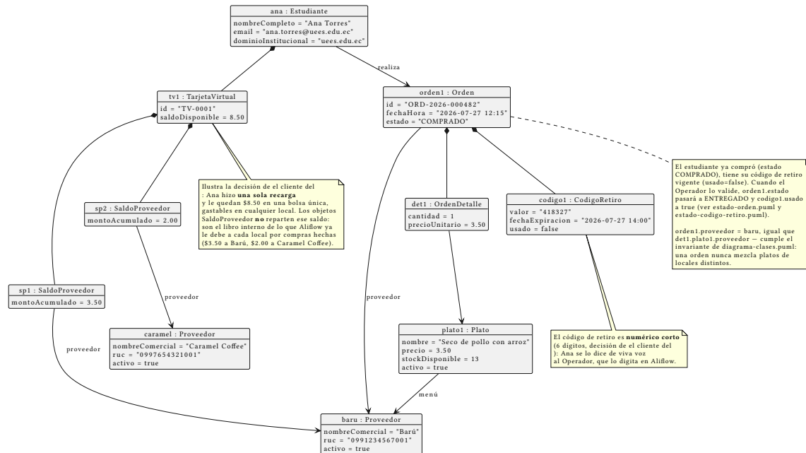
Figura 7: Diagrama de objetos: billetera y orden
