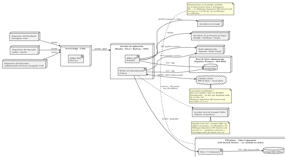
Figura 10: Diagrama de despliegue de Aliflow
